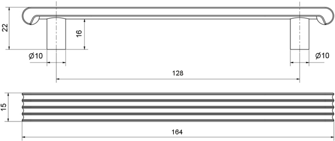
PC2990-128
