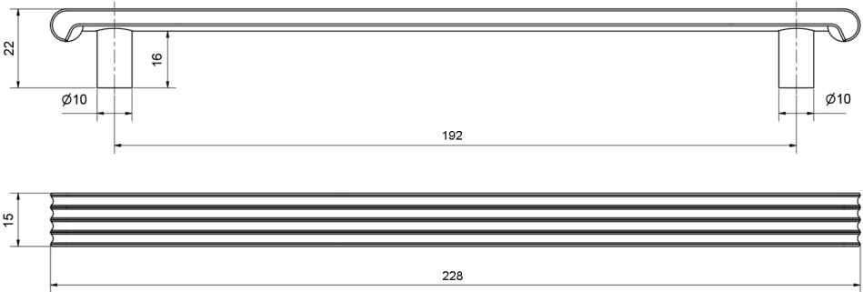
PC2990-192
